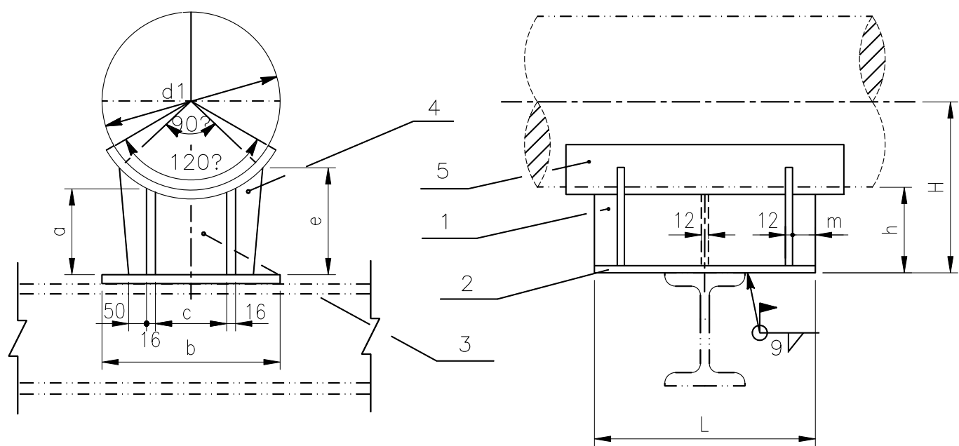
ELEV.
