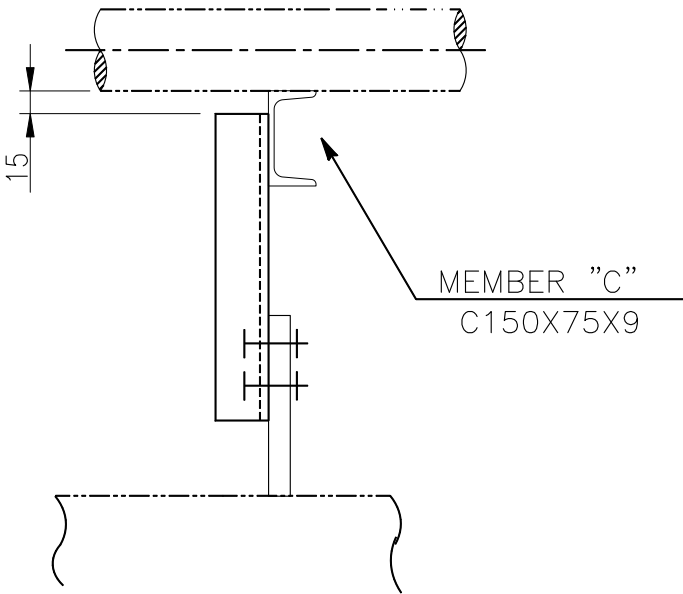
ELEV.
