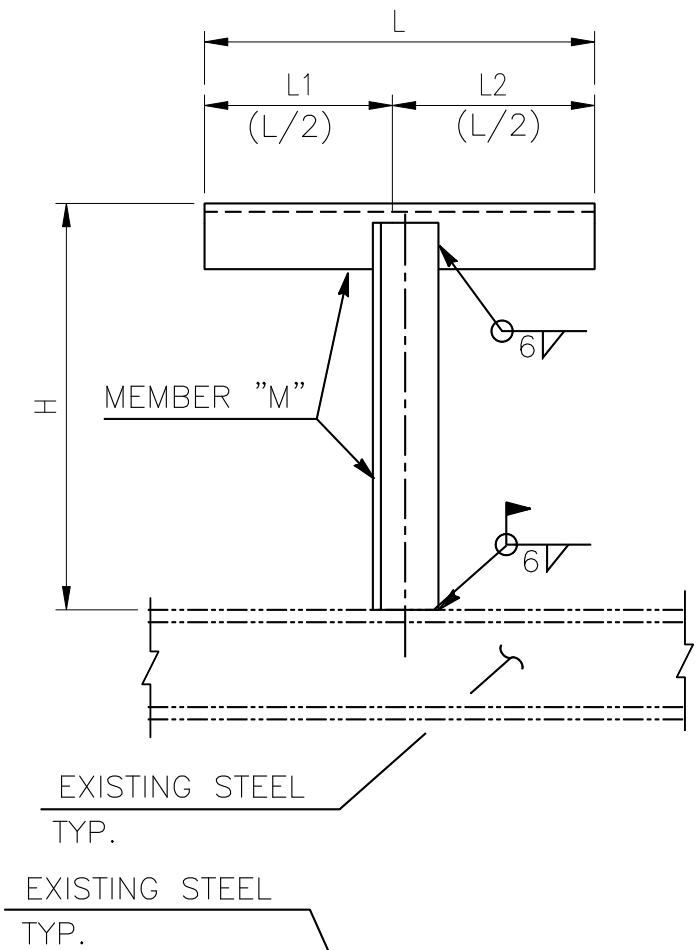
FIG.-A (ELEV.)
