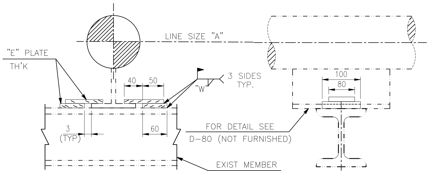
FIG. A
